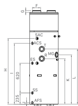
VISTA TRASERA HYDREA 280
