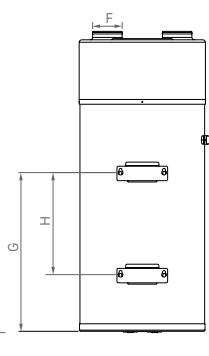
VISTA TRASERA HYDREA 150
