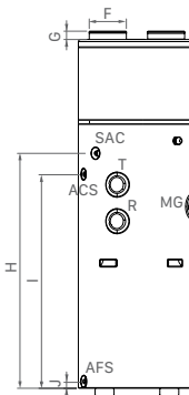
VISTA TRASERA HYDREA 200
