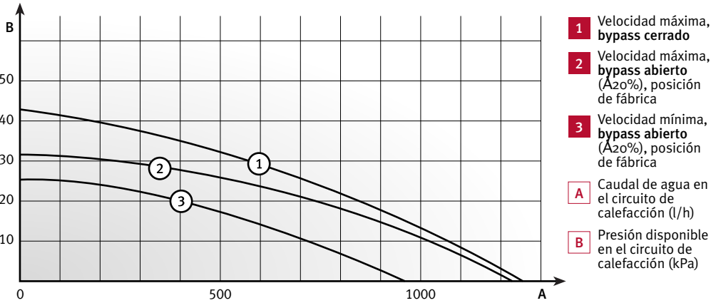
Curva de presión disponible de la bomba del circuito de calefacción Duomax Condens de 34/90 L
